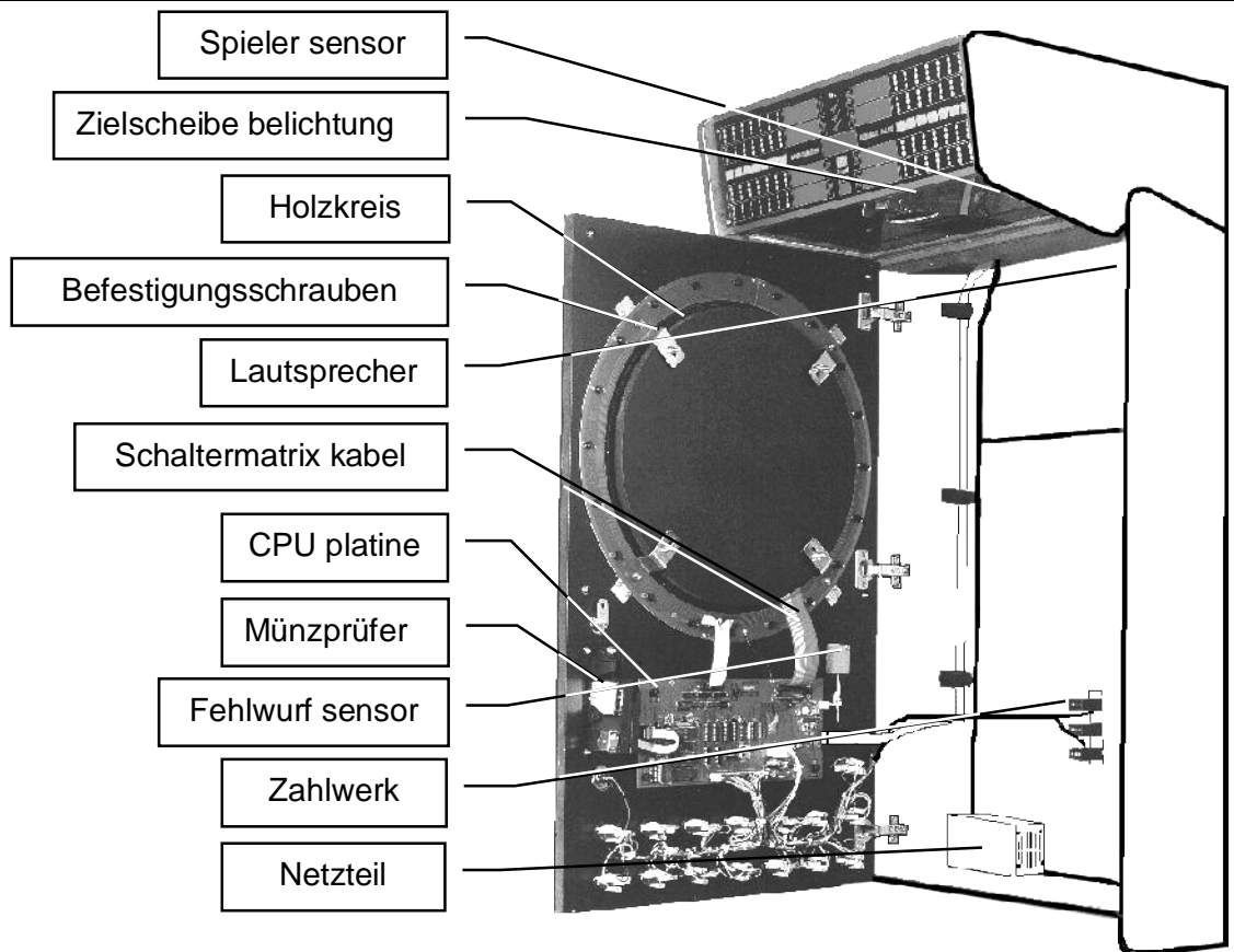
Abb.3 Aussehen des Inneren des Apparates
